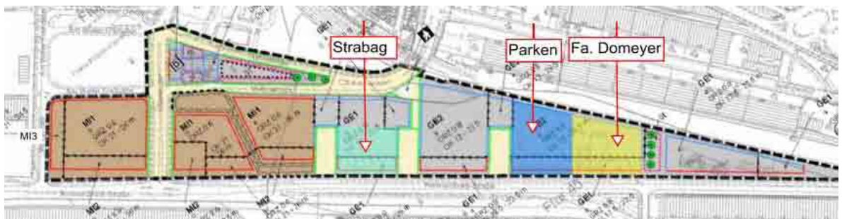
Abb. 32 Auszug aus dem Bebauungsplanentwurf 2409
