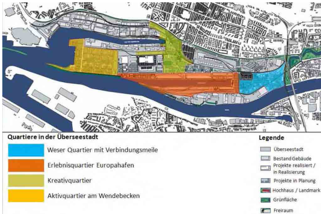
Abb. 7 Quartiere in der Überseestadt
